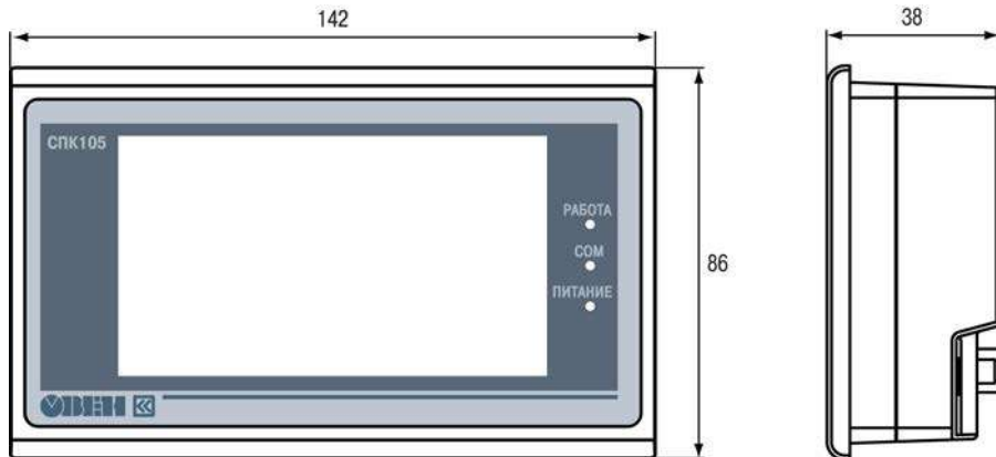
Рисунок А.1 – Габаритные размеры СПК105
